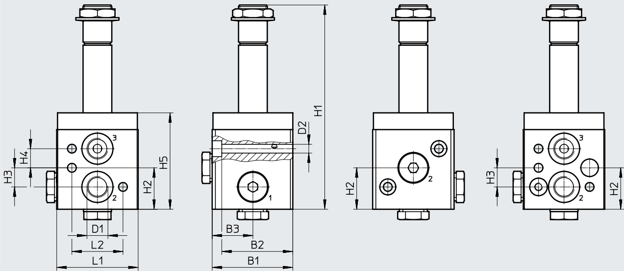
尺寸 – G1/4 基本阀和 NAMUR
