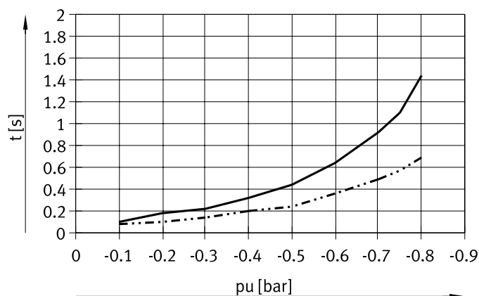
6 bar 工作压力时, 抽气时间 t 与 1 l 容积真空度 p_u 的关系
