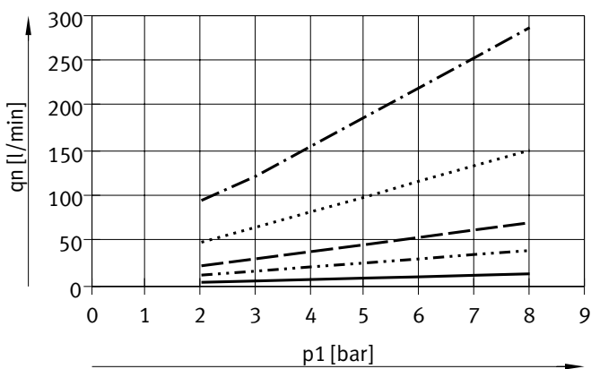
耗气量 q_n 与工作压力 p_1 的关系 高真空度/大抽气量
