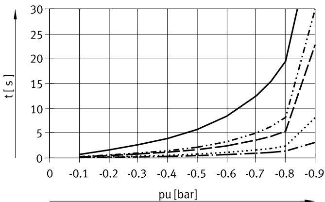
6 bar 工作压力时, 抽气时间 t 与 1 l 容积真空度 p_u 的关系 高真空度
