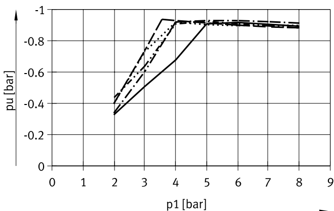
真空度 p_u 与工作压力 p_1 的关系 高真空度
