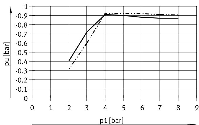
真空度 p_u 与工作压力 p_1 的关系
