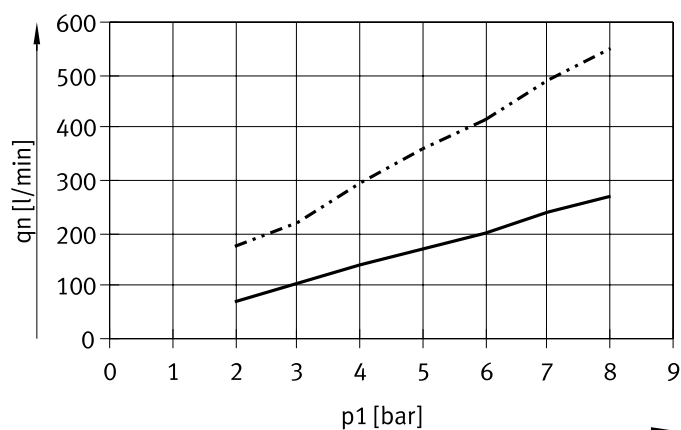
耗气量 q_n 与工作压力 p_1 的关系
