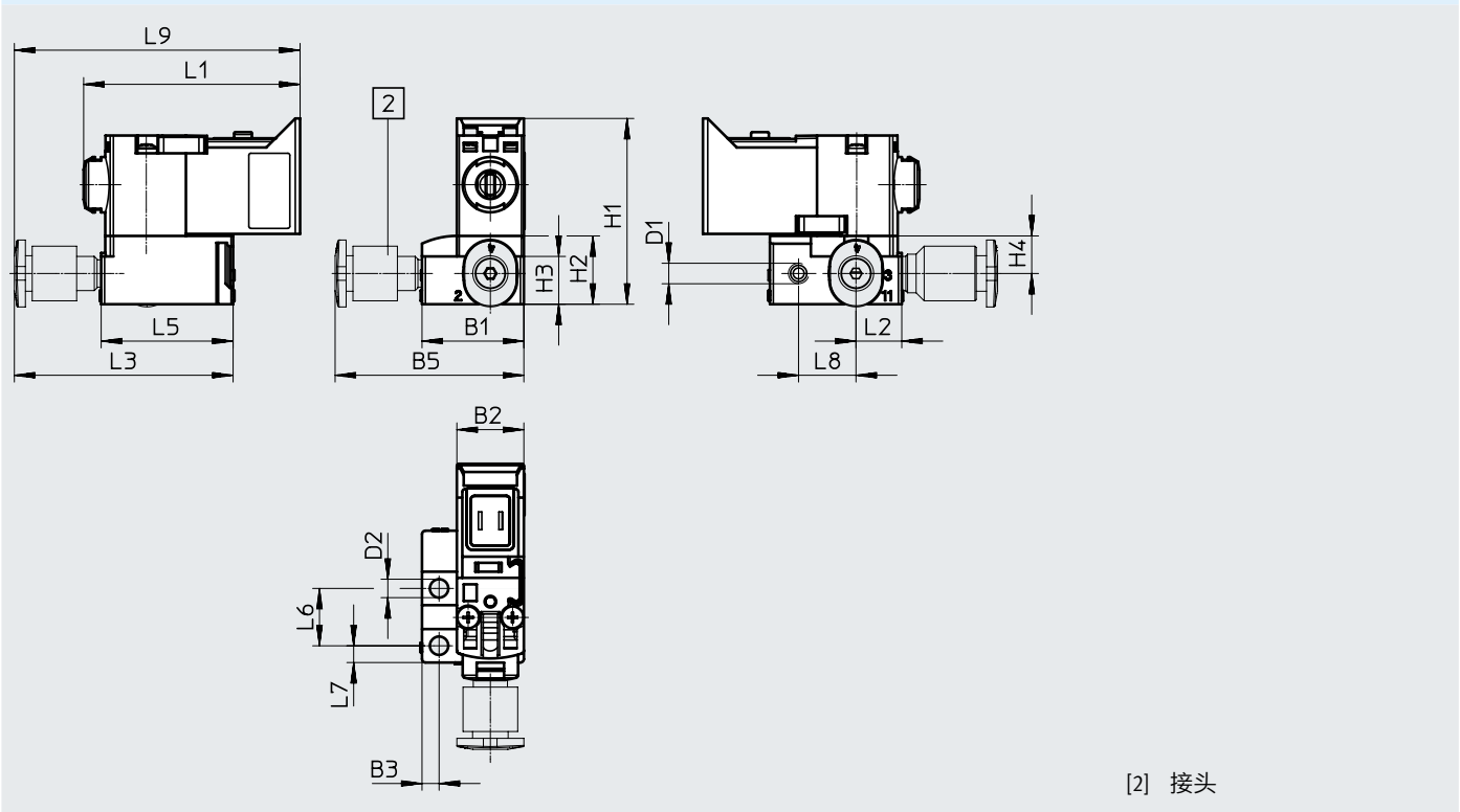
尺寸 - 单个底座上安装
