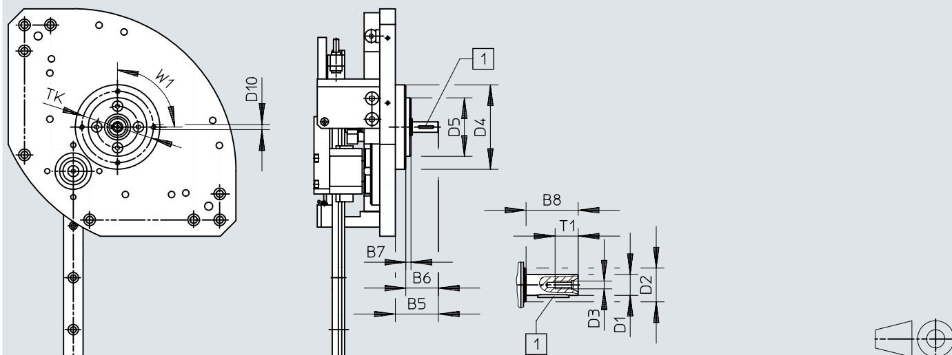
Dimensions – HSW-...-AS
