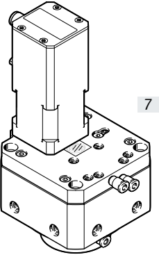
能源贯穿连接，气动
