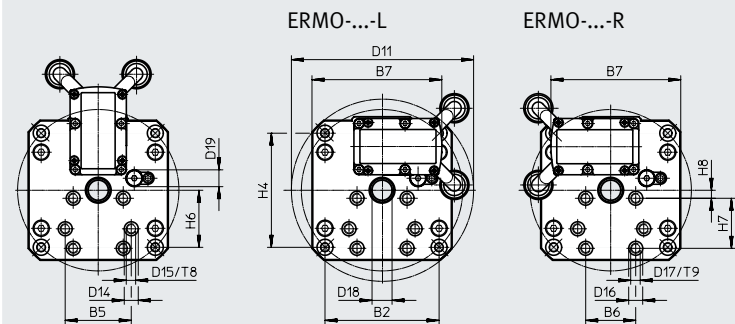
视图 A
