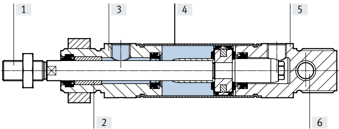
剖面图
