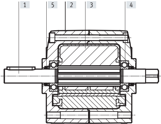
DRVS-12 ... 40
