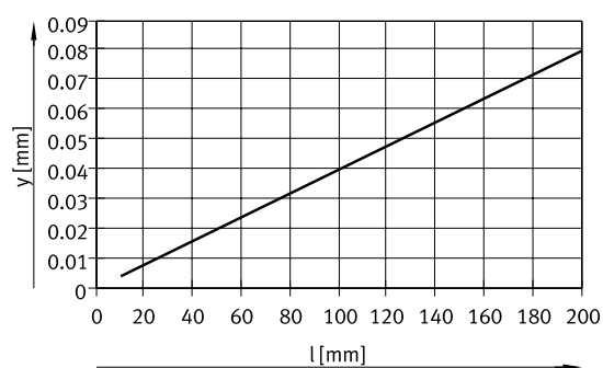
直线行程精度 y 与行程长度 l 的关系
