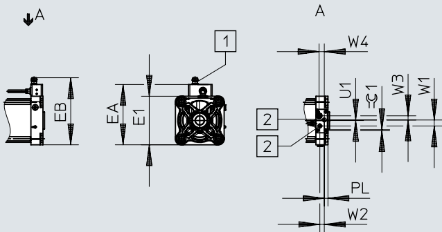
Dimensions – Variants DFPI-...-E-NB3P9B2-... and DFPI-...-E-NB3M12B2-...
