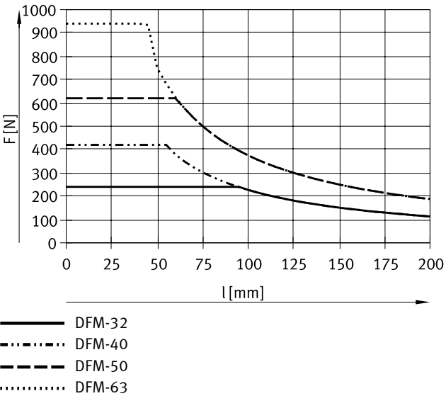
DFM-32 ... 63-GF, 行程 80 ... 100 mm
