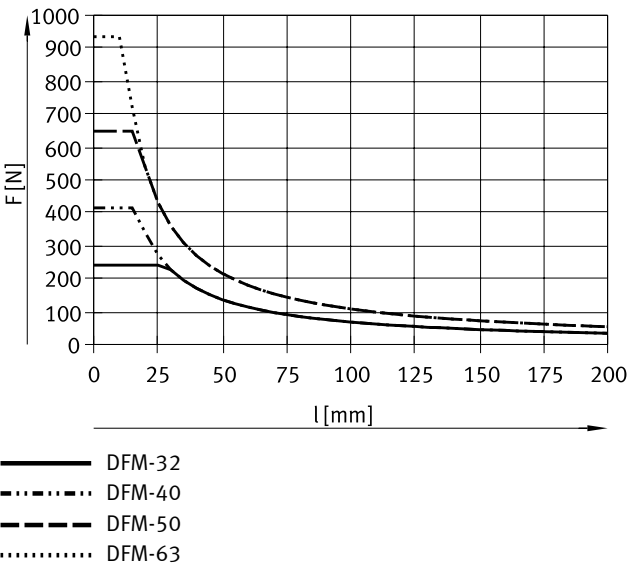
DFM-32 ... 63-KF, 行程最高可达 50 mm
