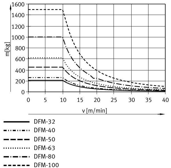
DFM-32 ... 100-GF, 行程 < 50 mm
