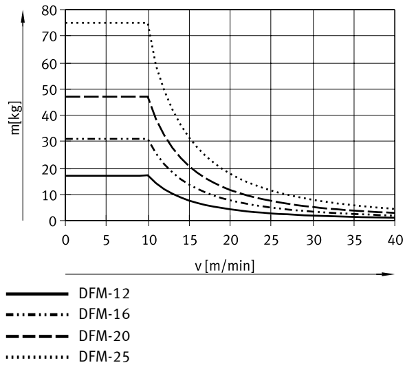
DFM-12 ... 25-GF, 行程 < 30 mm
