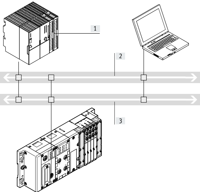
[1] 上位控制器 (PLC) [2] 现场总线 [3] IT 服务:
