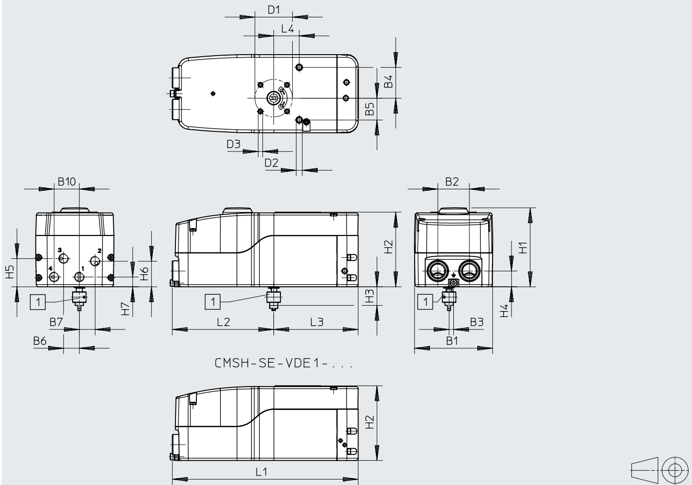
[1] 联轴器 CAFM-M1-CK-N1
