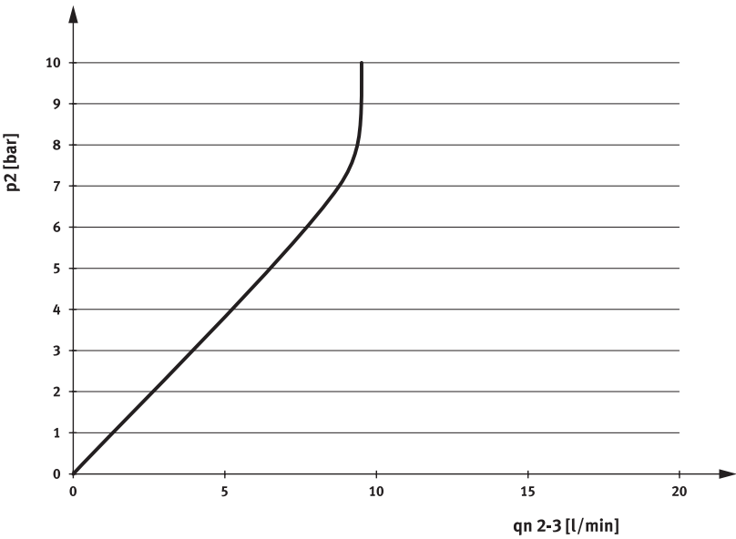
流量2→3qn時の出力圧力p2
