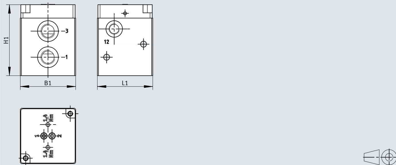
Dimensions – VOFC-LT-...G14-P2
