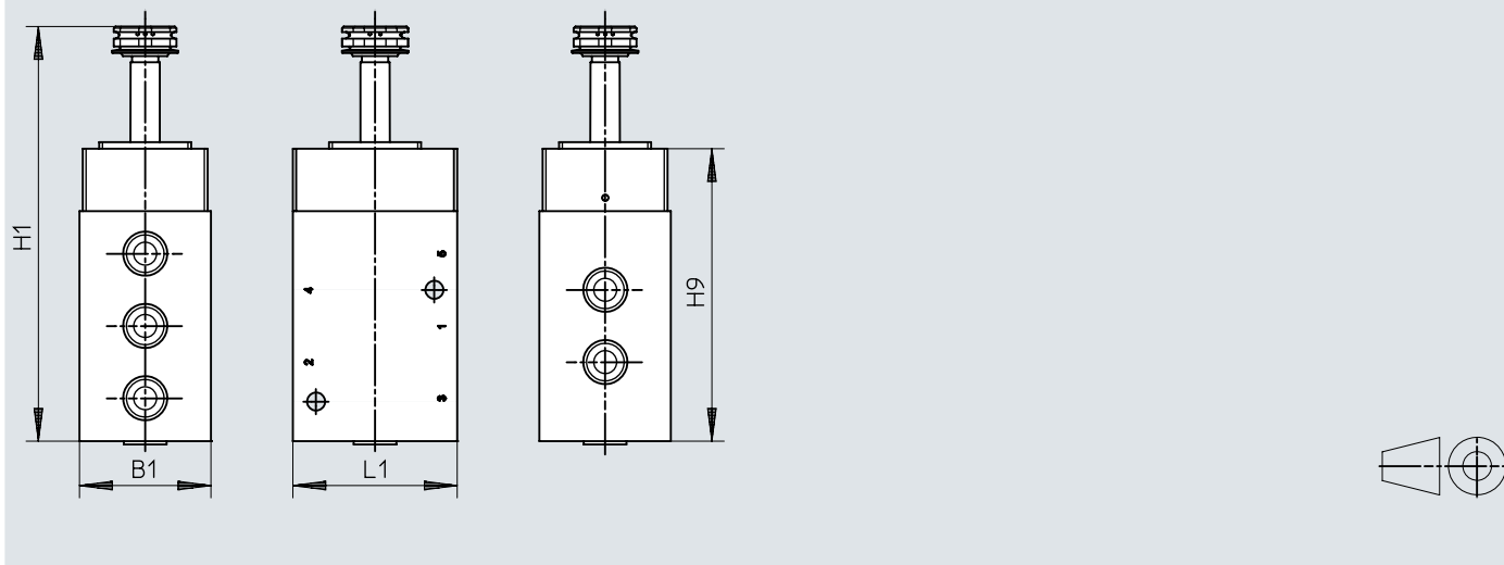
Dimensions – VOFC-L-...-FN
