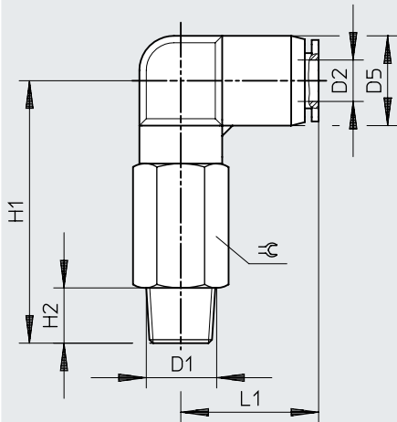
Dimensiones – Racor rápido roscado en L (largo), QBLL
