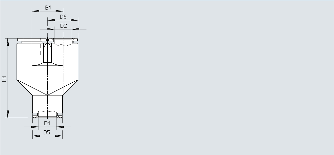
Dimensiones – Unión rápida en Y NPQH-Y, reductor
