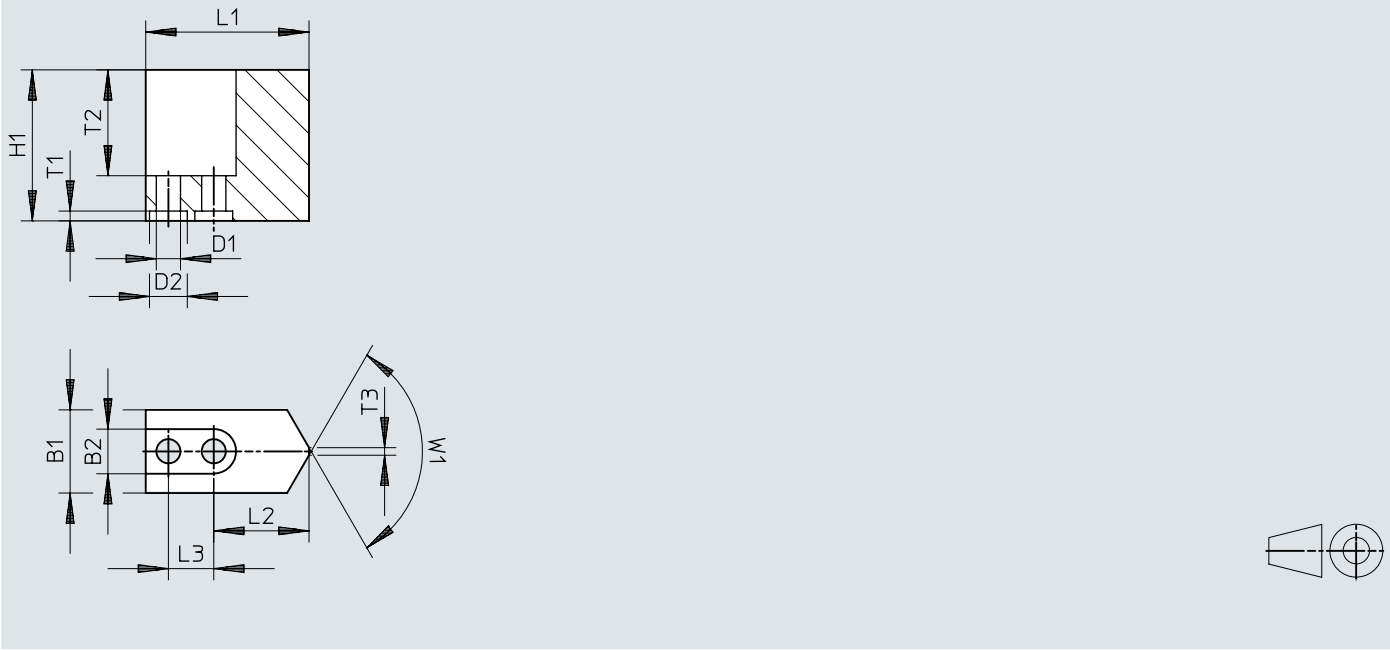
Dimensiones – Pinza de mandíbula adaptable BUB-HGDT-25
