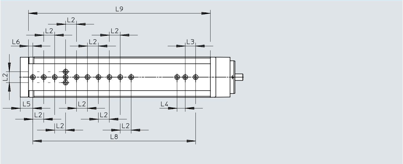
Dimensions – EGSL-75-200
