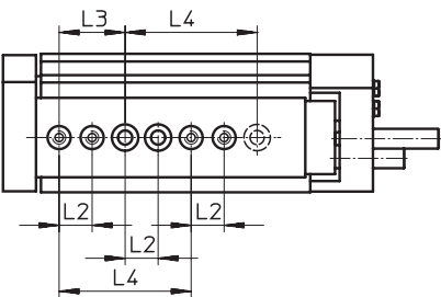
DGSL-8-30
