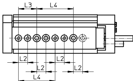
DGSL-10-30
