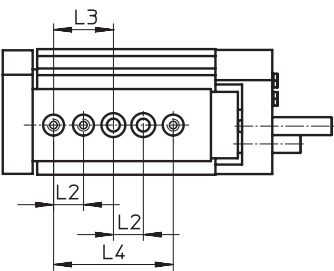
DGSL-8-30
