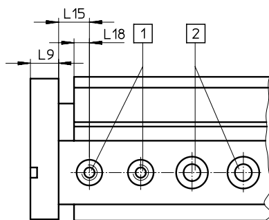
DGSL-4 ... 10
