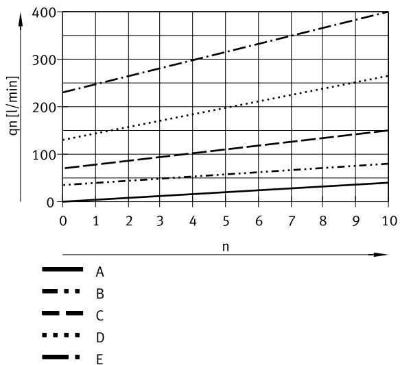
Normaldurchfluss q_n bei 6 → 0 bar in Abhängigkeit der Stellung Drosselschraube (Skala) n (GRLSA-1/8 – Steckanschluss QS, Metall)
