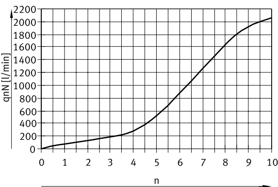
Normalnenndurchfluss qnN bei 6 → 5 bar in Abhängigkeit der Spindelumdrehungen n (GRLA/GRLZ-1/2 – Innengewinde/Stecknippel, Metall)
