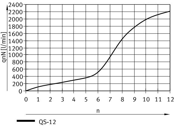
Normaldurchfluss qn bei 6 → 0 bar in Abhängigkeit der Spindelumdrehungen n (GRLA/GRLZ-1/2 – Steckanschluss QS, Metall)
