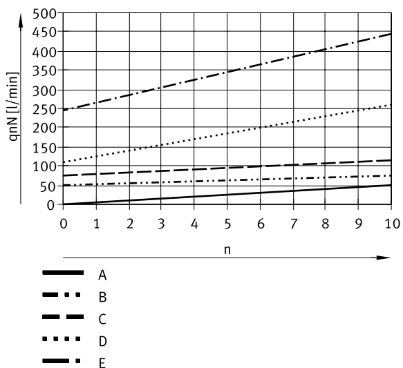
Normalenndurchfluss q_{nN} bei 6 → 5 bar in Abhängigkeit der Stellung Drosselschraube (Skala) n (GRLSA-1/4 – Steckanschluss QS, Metall)
