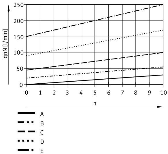
Normalenndurchfluss q_{nN} bei 6 → 5 bar in Abhängigkeit der Stellung Drosselschraube (Skala) n (GRLSA-1/8 – Steckanschluss QS, Metall)
