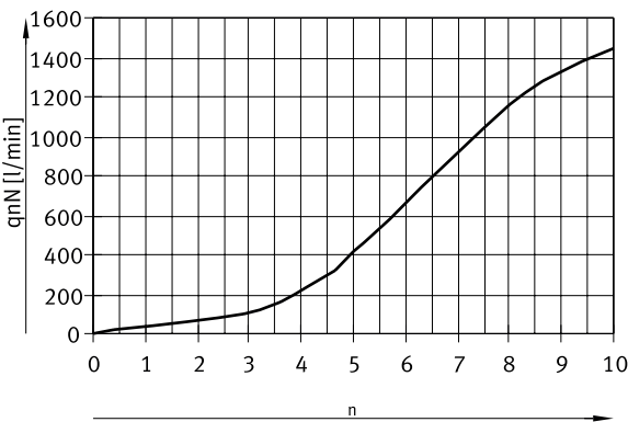
Normalnenndurchfluss qnN bei 6 → 5 bar in Abhängigkeit der Spindelumdrehungen n (GRLA/GRLZ-3/8 – Innengewinde/Stecknippel, Metall)
