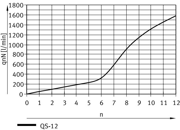
Normalnennendurchfluss qnN bei 6 → 5 bar in Abhängigkeit der Spindelumdrehungen n (GRLA/GRLZ-1/2 – Steckanschluss QS, Metall)
