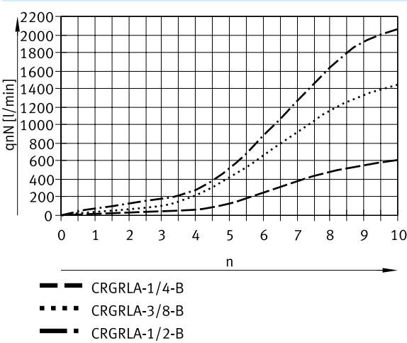
Normalnennendurchfluss qnN bei 6 → 5 bar in Abhängigkeit der Spindelumdrehungen n (CRGRLA-1/4, CRGRLA-3/8, CRGRLA-1/2 – Innengewinde, Edelstahl)
