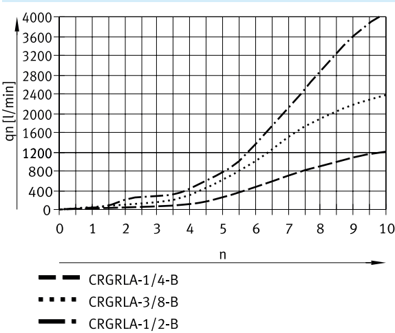
Normaldurchfluss qn bei 6 → 0 bar in Abhängigkeit der Spindelumdrehungen n (CRGRLA-1/4, CRGRLA-3/8, CRGRLA-1/2 – Innengewinde, Edelstahl)
