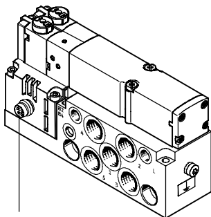
Connecteur mâle M8 x 1 à 4 pôles selon EN 60 947-5-2
