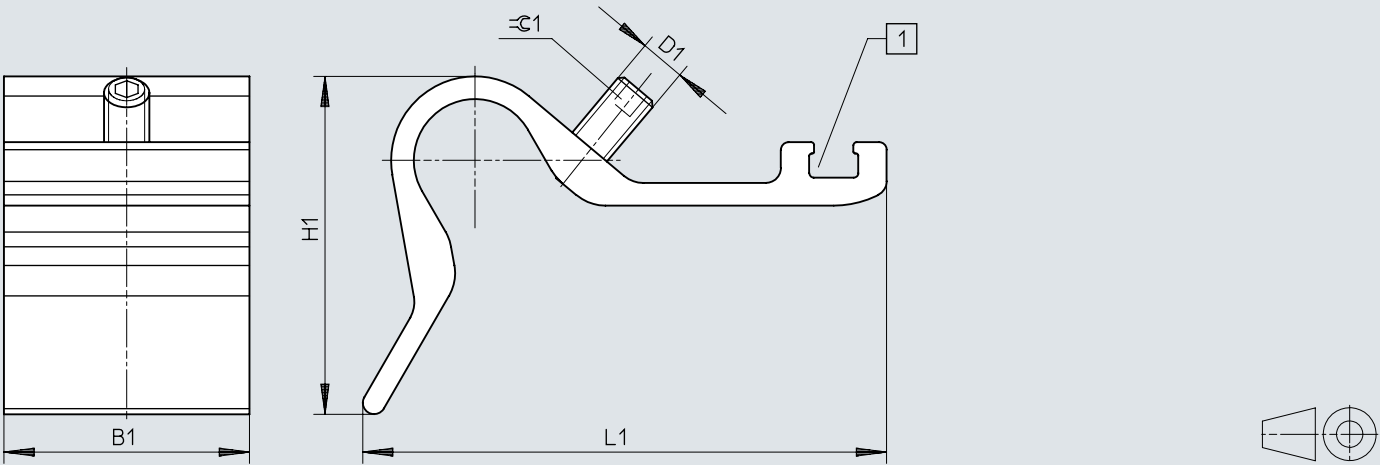
Dimensiones – Soporte para sensor DASP-M4-...-A
