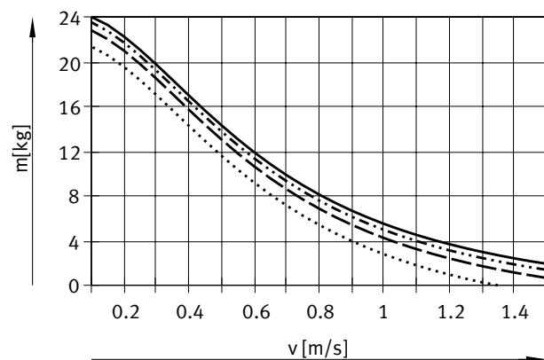
DFM-32-...-B-YSRW
