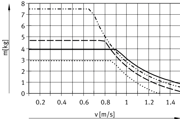
DFM-20-...-B-YSRW
