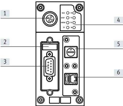
Pin allocation – CPX-CEC-C1/-M1
