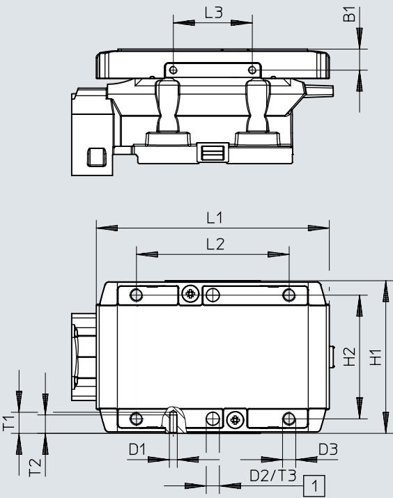
[1] Bohrung für Zentrierhülse ZBH
