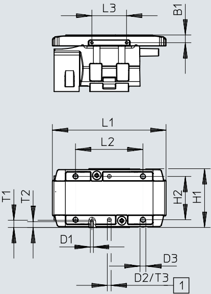
[1] Bohrung für Zentrierstift ZBS
