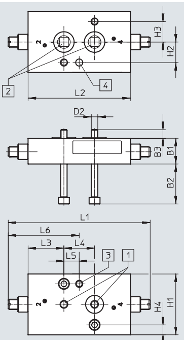
Double-acting VABF-...P2
