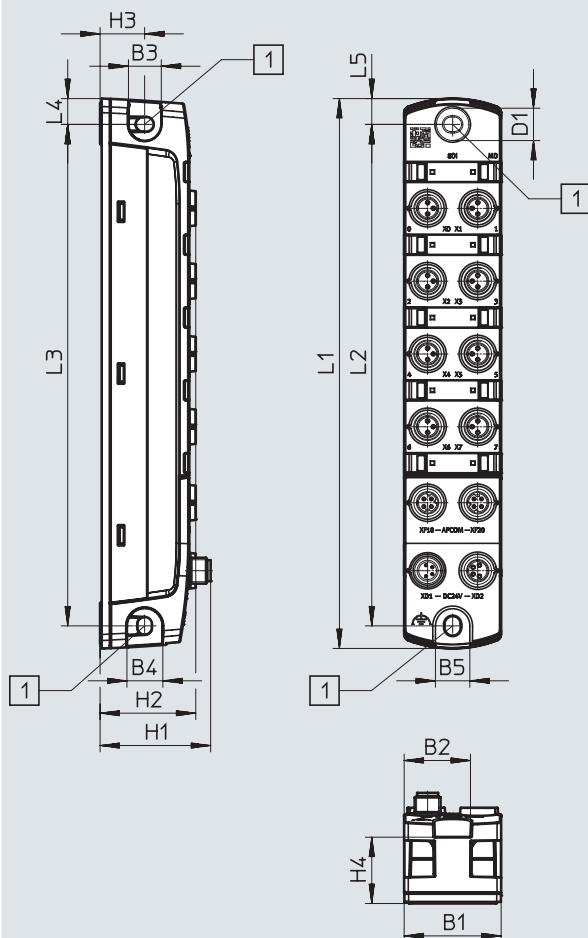
CPX-AP-I-8DI-M8-3P
