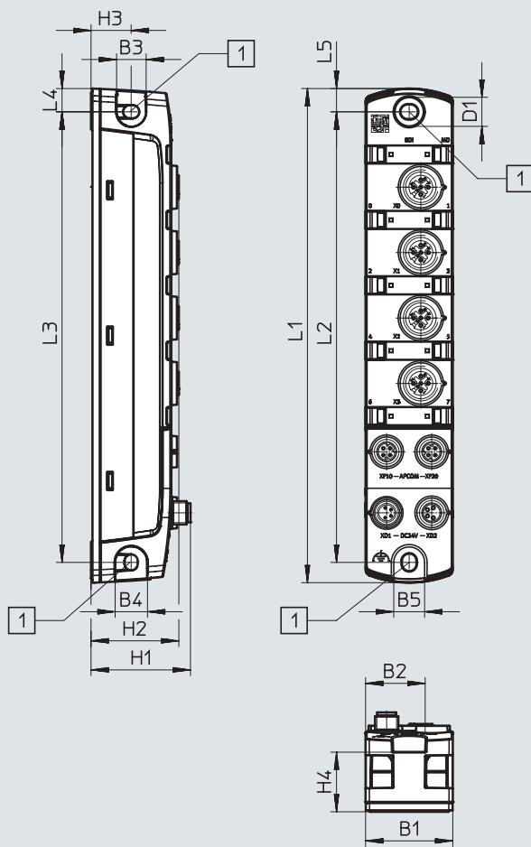
CPX-AP-I-8DI-M12-5P
