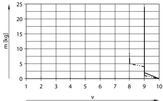
Masa m en función del nivel de velocidad v con conjunto paralelo EPCS-BS-32-3P EPCS-BS-32-8P
