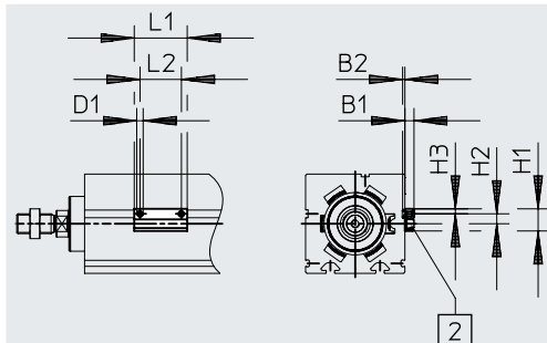
[2] Sensor de proximidad
