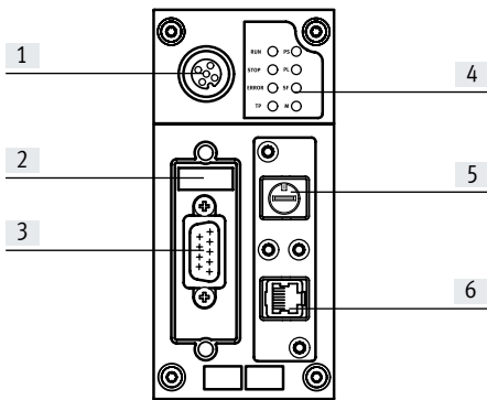
Asignación de pines – CPX-CEC-C1/-M1
