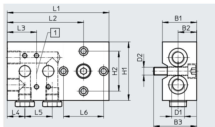
[1] NAMUR-Flansch
