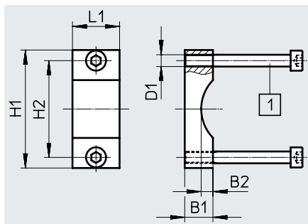
[1] Zylinderschraube, 2 Stück M5x45 und 2 Stück M5x65
