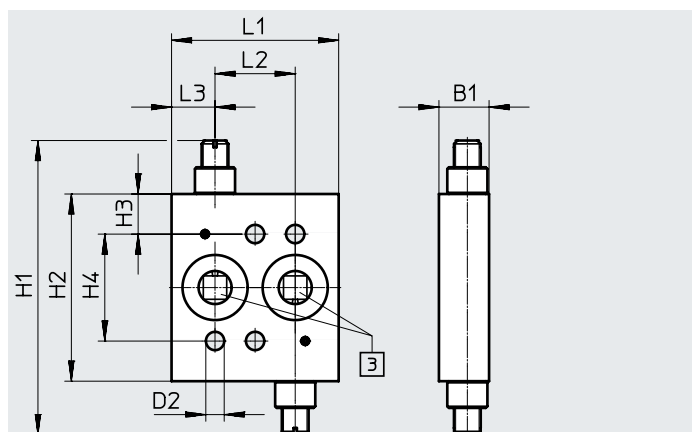
[1] Arbeitsanschlüsse für G1/4 und 1/4 NPT Ventile
