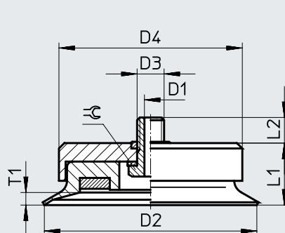
ESS-80/100-E
