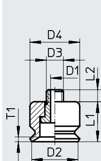
ESS-15-E
