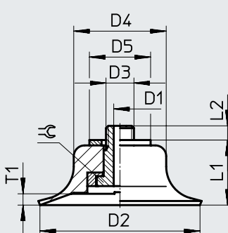
ESS-40/50/60-E
