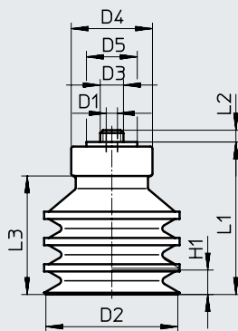
ESS-40/50-C
