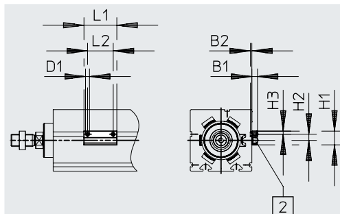
[2] Näherungsschalter
