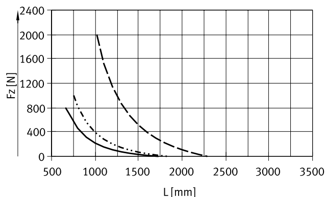
Kraft F_z
