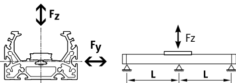
Kraft Fz
