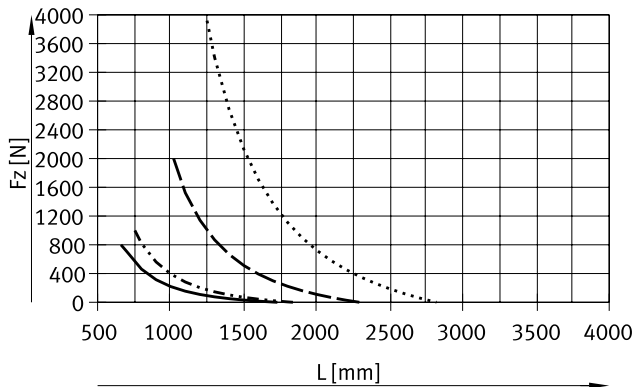
Kraft Fz
