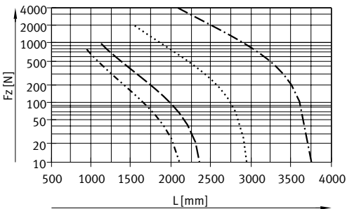
Kraft Fz
