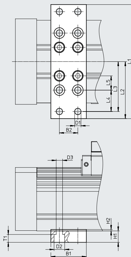
Baugröße 120
