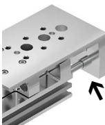
[6] Spielfreie Kolbenstangen/Jochanbindung
