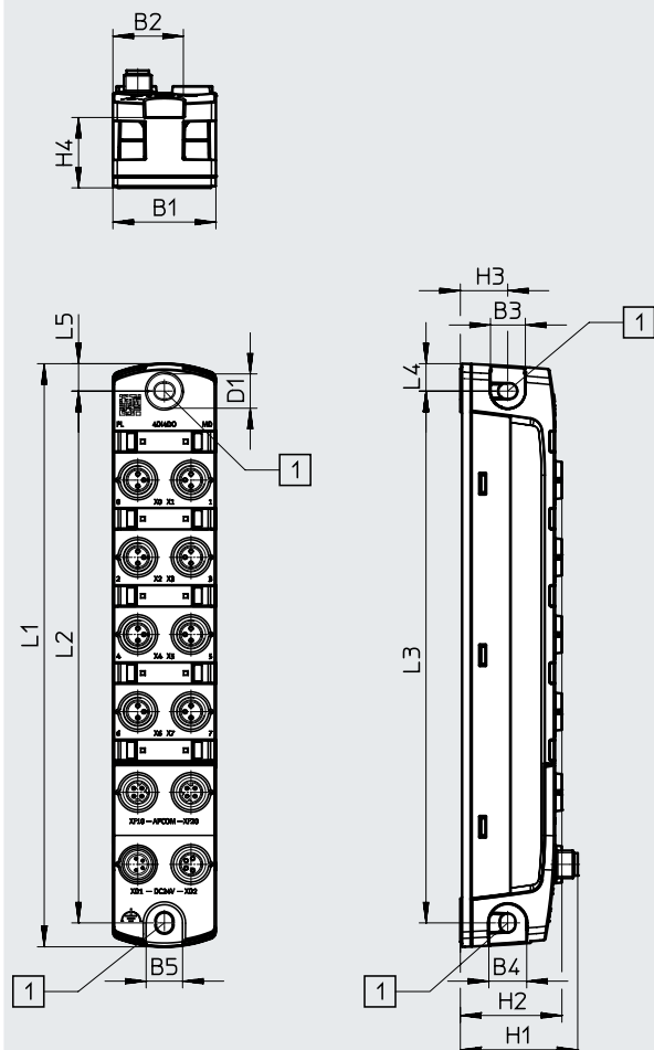
CPX-AP-I-4DI4DO-M8-3P
