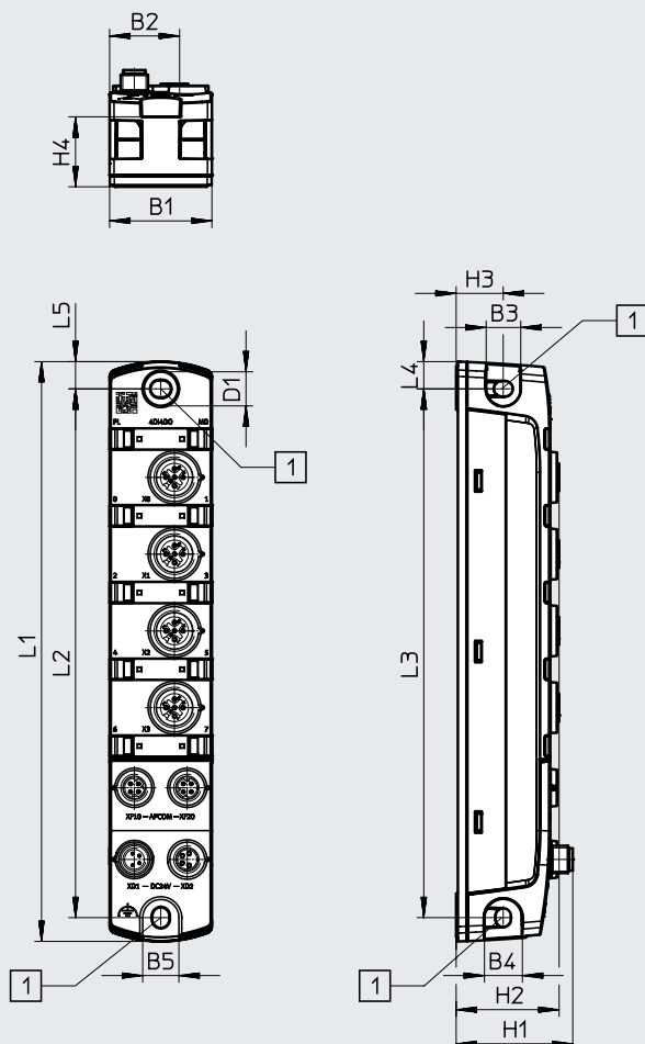
CPX-AP-I-4DI4DO-M12-5P
