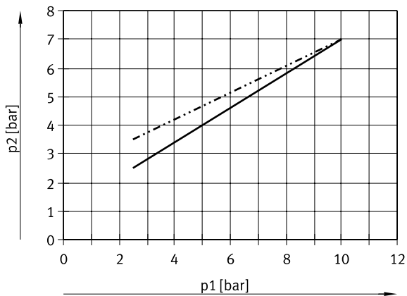
Tamaño 30: presión de mando p2 en función de la presión de trabajo p1 con alimentación externa del aire de pilotaje
