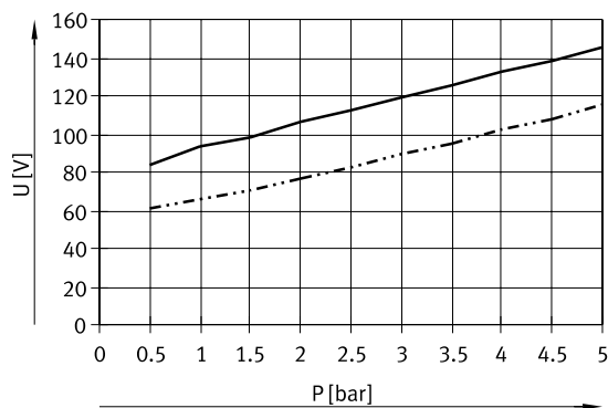
Tensión para abrir y cerrar la válvula en función de una presión de funcionamiento con 300 V
