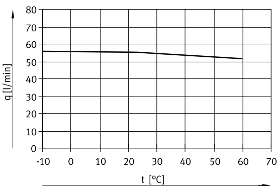
Caudal qn en función de la temperatura ambiente con 300 V
