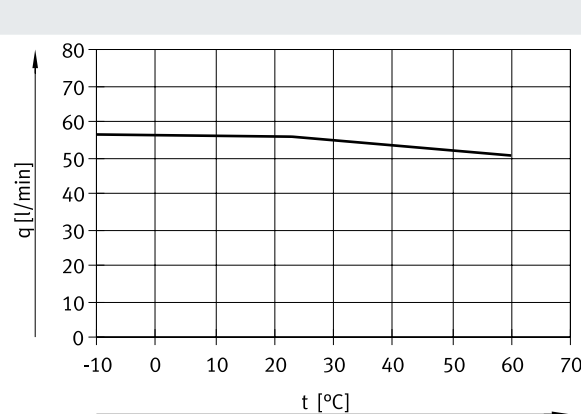
Caudal qn en función de la temperatura ambiente con 300 V
