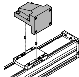
Con conjunto de sujeción angular EHAA-D-L2-...-AP
