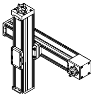
Matriz de combinaciones entre eje ELGC/ELGS-TB, ELGC/ELGS-BS, minicarro EGSC/EGSS-BS, cilindro eléctrico EPCC/EPCS-BS y eje de guía pasiva ELFC Opciones de montaje con con kit adaptador o fijación directa
