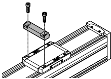
Con fijación para perfil EAHF-L2-...-P-D...
