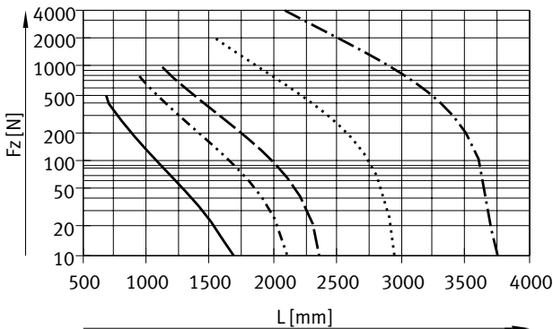
Fuerza F_z
