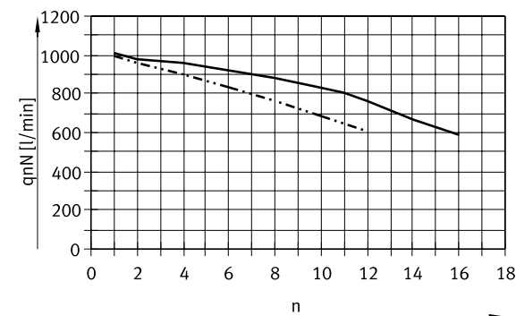
Baugröße 25 – Normalnenndurchfluss qnN, bei mehreren zeitgleich geschalteten Ventilen n für 3/2-Wegeventile für 5/2-, und 5/3-Wegeventile
