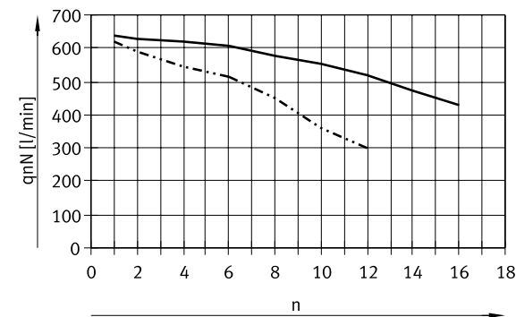
Baugröße 20 – Normalnenndurchfluss qnN, bei mehreren zeitgleich geschalteten Ventilen n für 3/2-Wegeventile für 5/2-, und 5/3-Wegeventile
