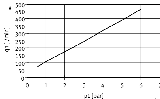
Luftverbrauch qn in Abhängigkeit vom Betriebsdruck p1
