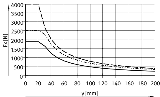
Max. Axialkraft Fx, statisch, drückend und ziehend
