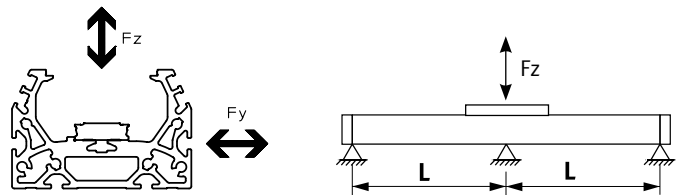
Kraft F_z
