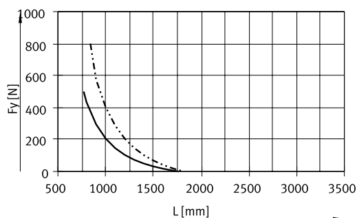
Kraft F_y
