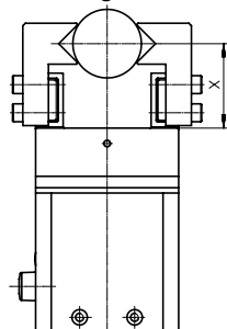
Einbaulage senkrecht
