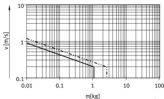
Kolben-Ø 8/12 mit YSR-Dämpfung
