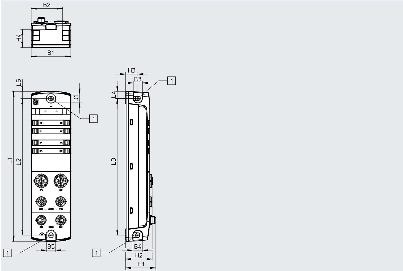
[1] Befestigungsbohrung für Schrauben M4
