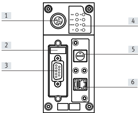
Pin allocation – CPX-CEC/CPX-CEC-S1-V3
