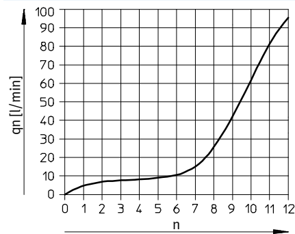
Normaldurchfluss q_n bei 6 bar \rightarrow 0 bar in Abhängigkeit der Spindelumdrehungen n GRLO/GRGO-M3
