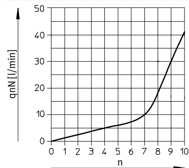
Normalnennendurchfluss q_{nN} bei 6 bar \rightarrow 5 bar in Abhängigkeit der Spindelumdrehungen n GRLO/GRGO-M3
