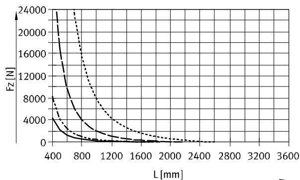
Kraft Fz
