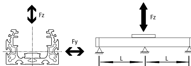
Kraft Fz
